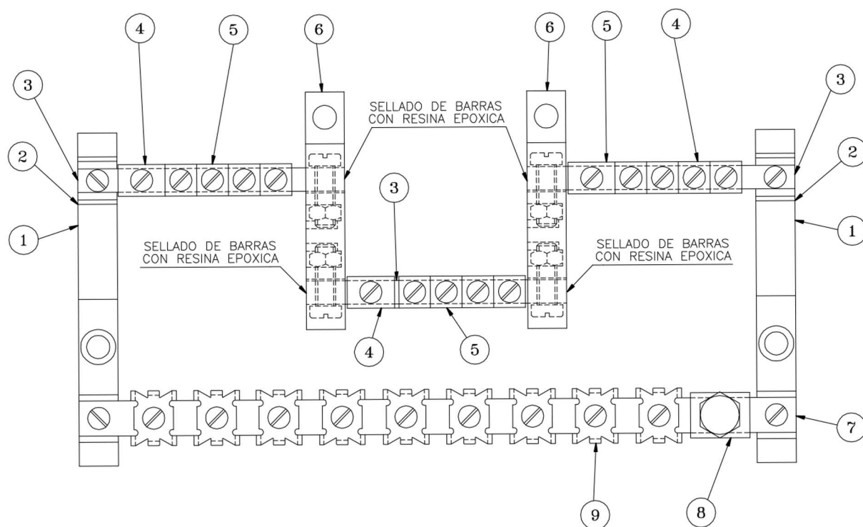
PLANTA DISPOSICIÓN GENERAL
