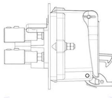
Hembra Empotrable 225-320
